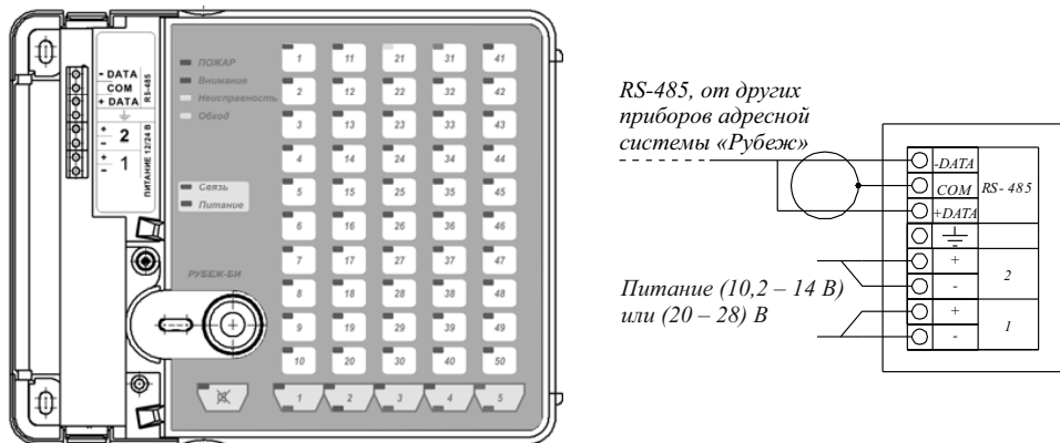
Рисунок 1 – Внешний вид и схема подключения прибора
